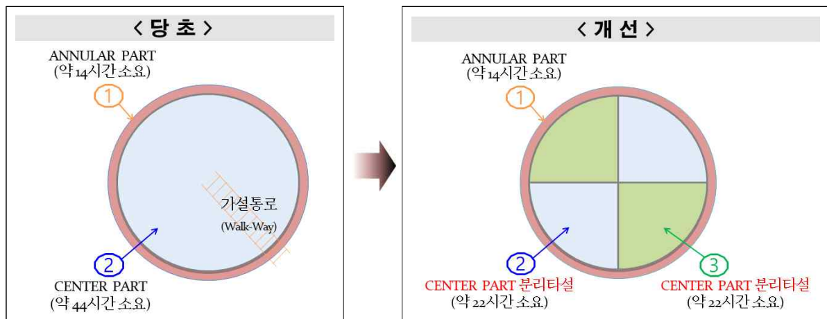
【그림 3】 바닥슬라브 콘크리트 분할타설 개선방안
