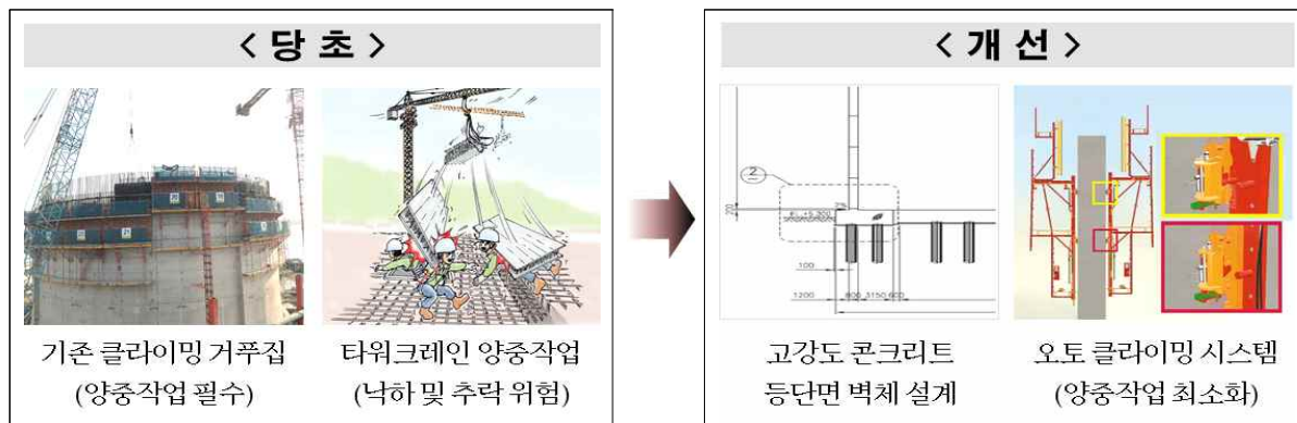
【그림 4】 저장탱크 벽체 거푸집 개선방안
